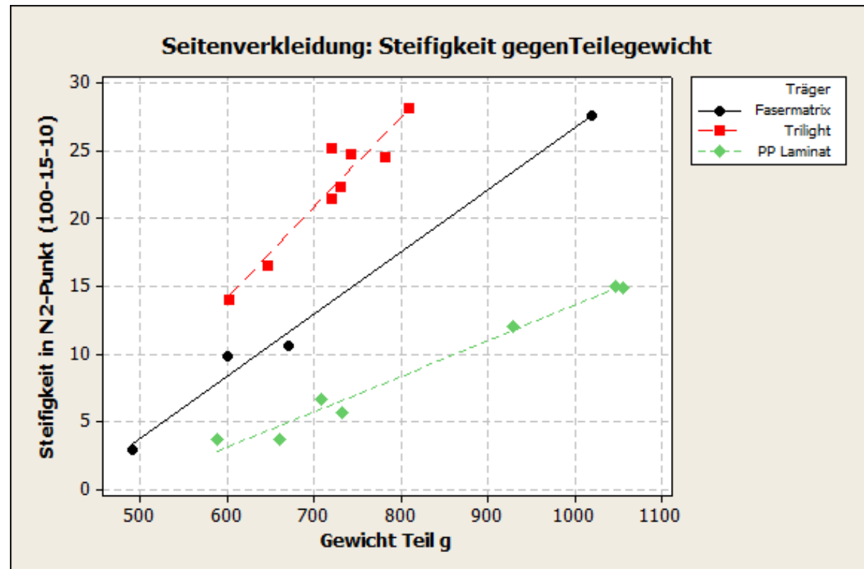
Modellversuch an einer Standard-Seitenverkleidung
